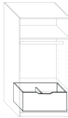
TIROIR POUR ARMOIRE 100 CM ART. 9536 H 39 x W 82 x D 46 CM
