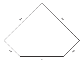
ARMOIRE D/ ANGLE PORTES COMPRISES ART. 565-10 H201 x W130 x D94 (POIGNÉES EXCLUES)
